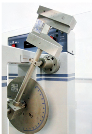
Figura 29. Equipo empleado para la determinación de impacto Charpy e Izod.
