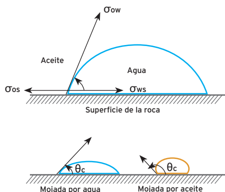
Figura 40. Representación esquemática de los ángulos implicados en el fenómeno de la tensión superficial de líquidos sobre superficies sólidas.
