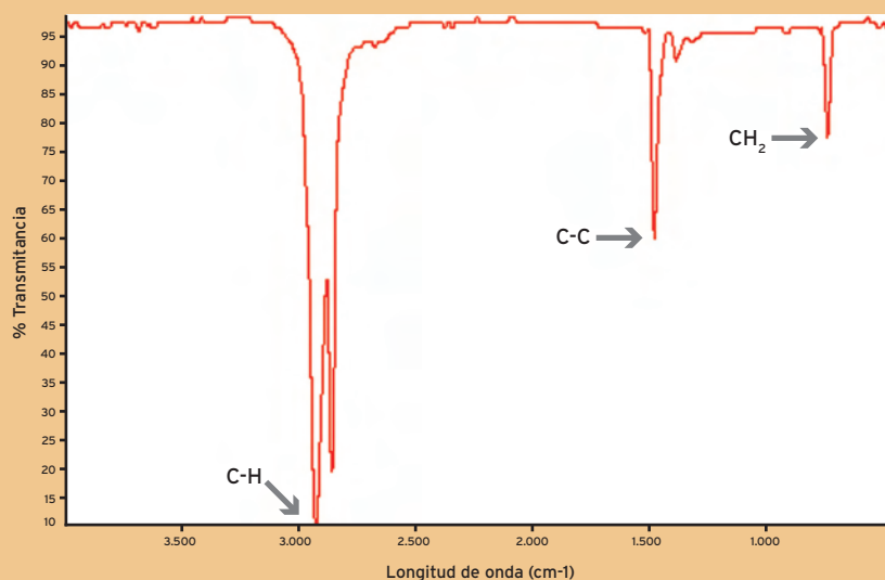
Figura 12. Espectro IR obtenido para una muestra de polietileno.
