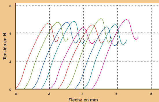
Figura 36. Gráfica tensión-deformación obtenida en ensayo de punción de film.
