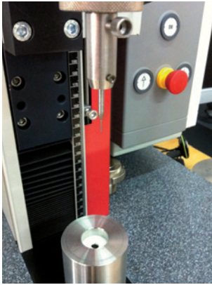
Figura 35. Fotografía de detalle del equipo de punción (por cortesía de Zwick/Roell).
