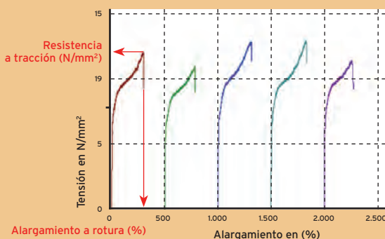
Figura 21. Ejemplo gráfica de resultados para un ensayo de tracción de film de 5 probetas.
